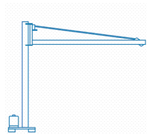
Säulenschwenkkran mit Mobilbodenplatte
