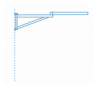
Wandschwenkkran mit Knickarmausleger
