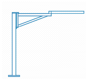
Säulenschwenkkran mit Knickarmausleger
