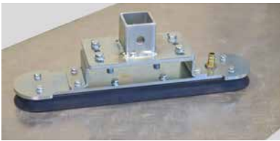
Ovale Saugplatte (für schmale Werkstücke und wenig Ansaugfläche)
