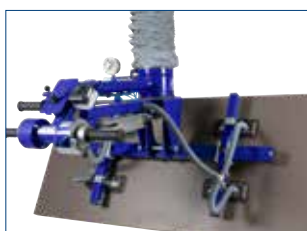
Plattenheber mit Schwenkvorrichtung (pne.)
